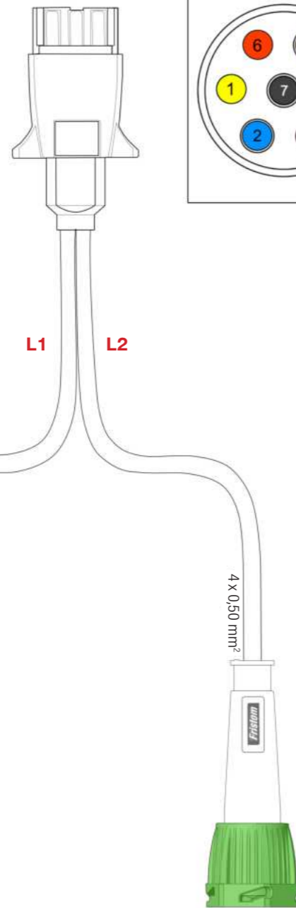
Plug 7 Pins Innerwork / Wtyk 7 Pinów Plug view / Widok od wtyczki / ISO 1724
