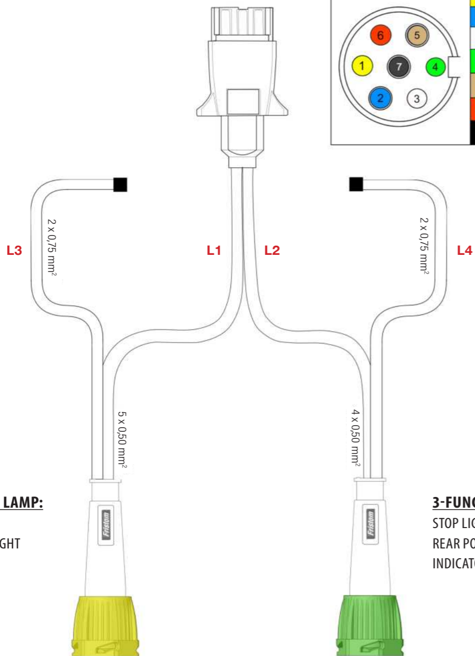
Plug 7 Pins Innerwork / Wtyk 7 Pinów Plug view / Widok od wtyczki / ISO 1724
