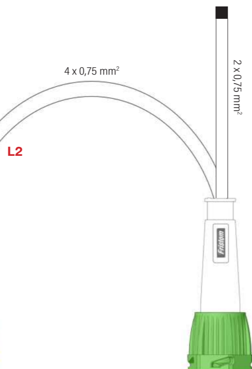
BAYONET 4 PIN Green / Zielony Plug view / Widok wtyczki
